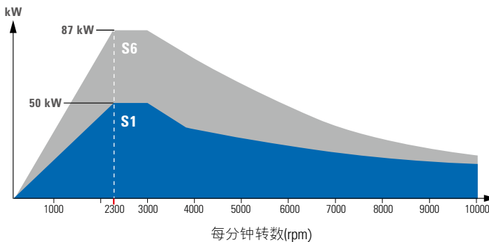
主轴功率
