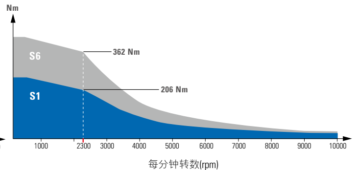
扭矩
